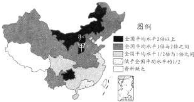
图 9 我国单位 GDP 二氧化碳排放量分布示意图
